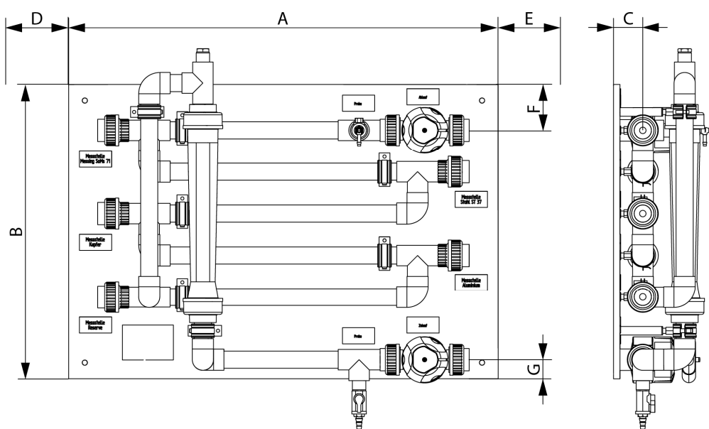
Abb. 2: Maßzeichnung
