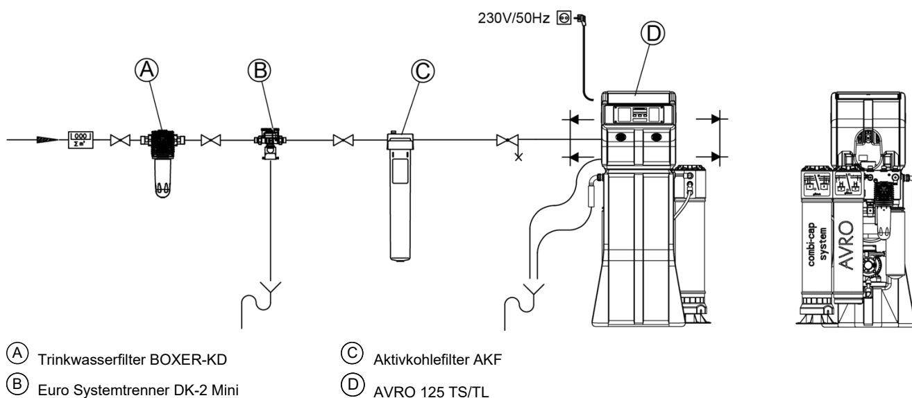
Abb. 2: Installationszeichnung
