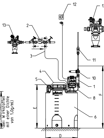
Abb.11.2: Einbauzeichnung DM-T 20 / DM-T 30
