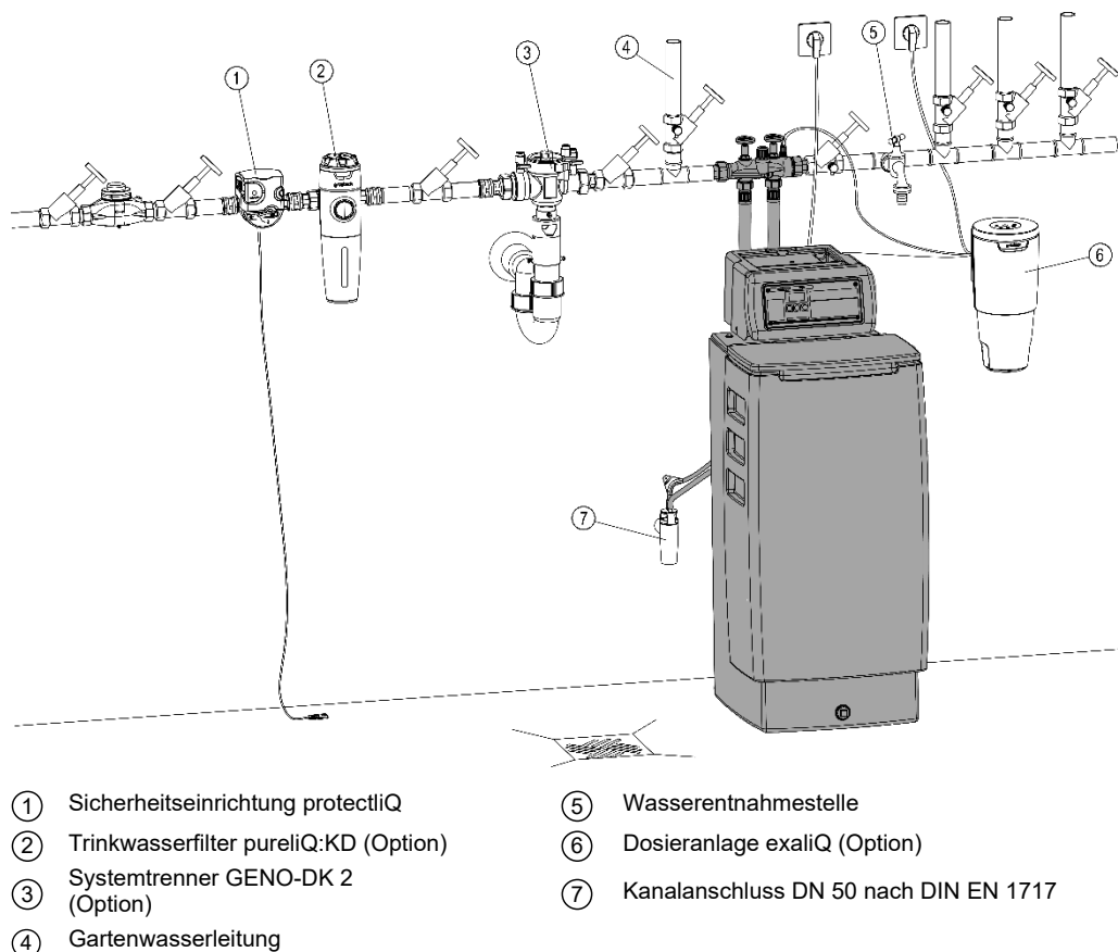
Abb. 3: Aufstellungszeichnung WINNI-mat VGX-N 400
