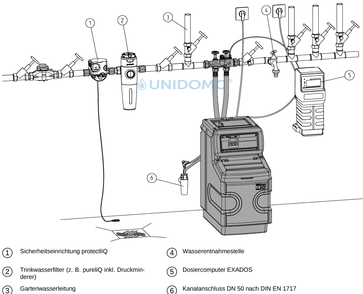
Abb. 2: Einbaubeispiel Enthärtungsanlage WINNI-mat VGX
