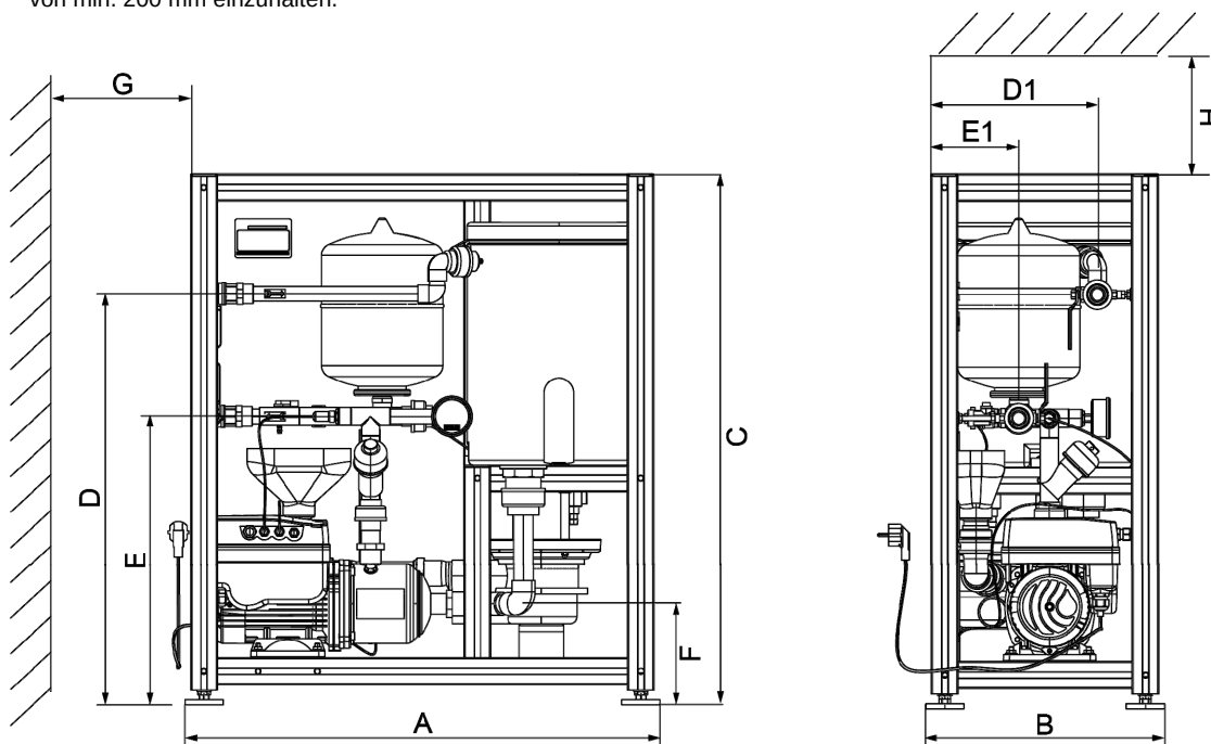
Abb.2: Maßzeichnung
