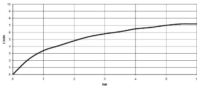
Durchflussdiagramm
