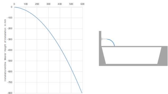
Wurfweitendiagramm
