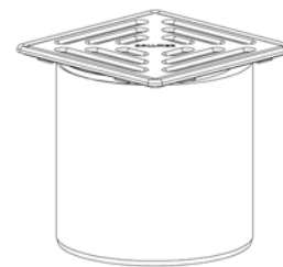
Aufsatz VEC 15, seitenverstellbar, 150 x 150 mm
