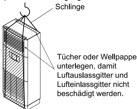
(2) Vertikale Aufhängung
