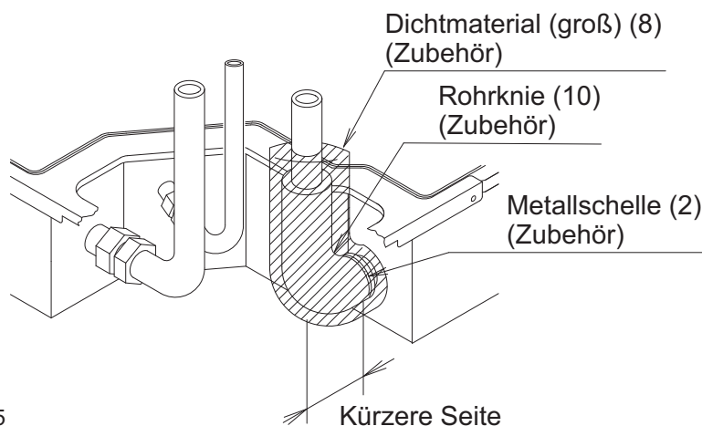
Abb. 25 (Aufsteigende Rohrleitung)
