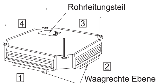
Fixiervorgang für Unterlegscheibe Abb. 16
