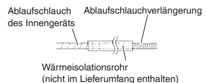
Ablaufschlauch mit dem Innengerät geliefert
