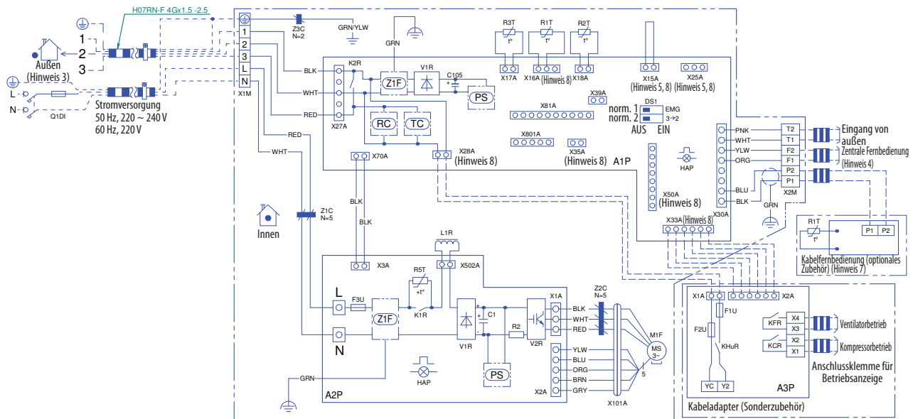
Schaltplan
