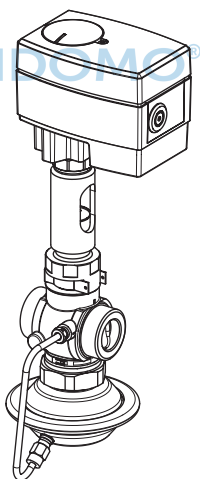
Adapter + AVQM + AMV(E) 10, 13
