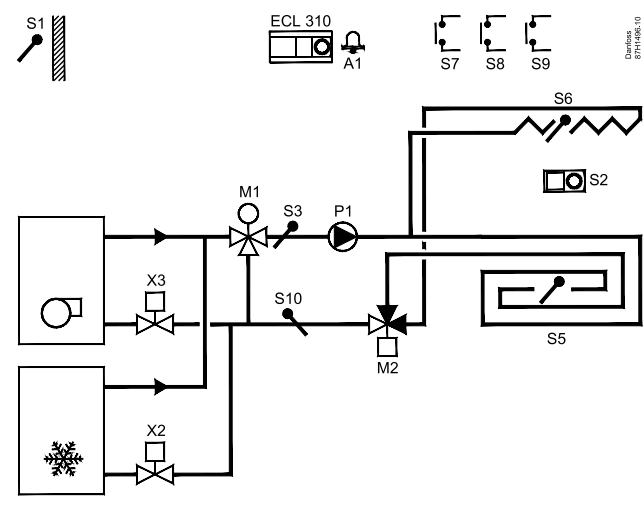
Typische A332.4-Applikation:
