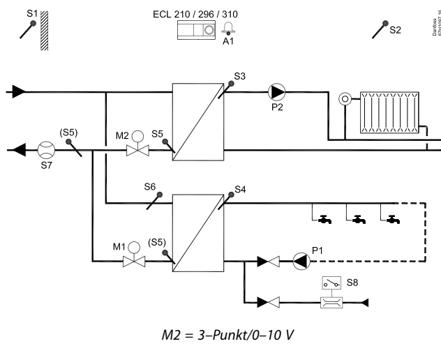
Typische A266.2-Applikation:
