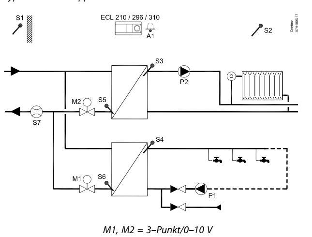
Typische A266.1-Applikation:
