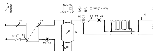
Typische A319.2-Applikation:
