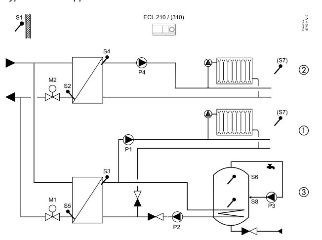
Typische A267-Applikation:
