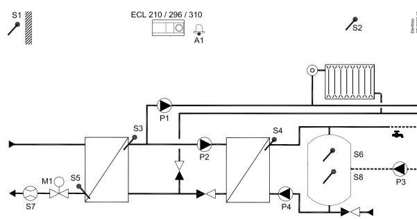
Typische A237.2/A337.2-Applikation:
