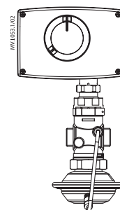
AMV 23, AMV 33 + AVQM (DN 15-50)
