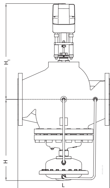
AMV 85, AMV 86 + AFQM (DN 150-250)
