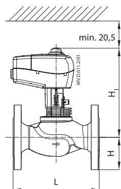
AME 335, AME 435 + VF 2, VL 2 (DN 15-80)
