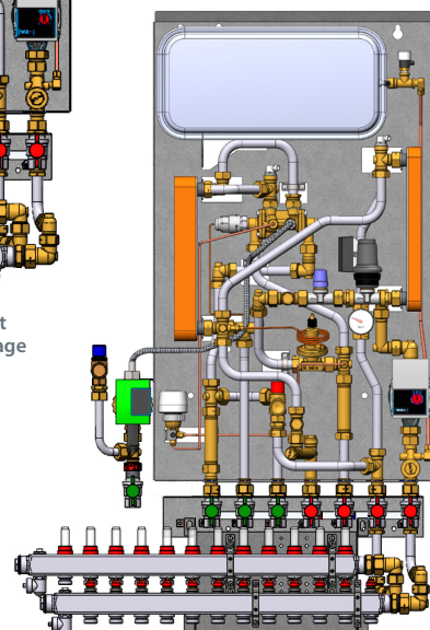
VX-F mit Montageschiene mit TWW-Zirkulationssatz-Montage und Verteilerstation mit 12 Heizkreisen
