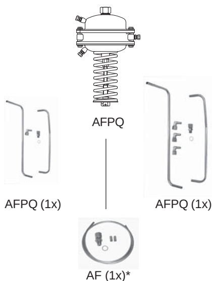
VFQ 2 (21) DN 15 - 125
