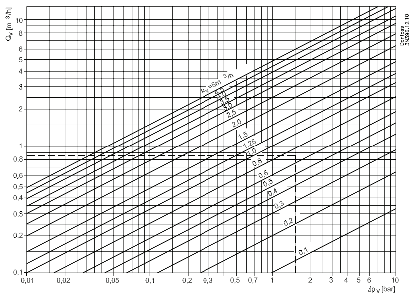
Abb.2 Abhängigkeit von Wassermenge und Druckabfall über dem Ventil.
