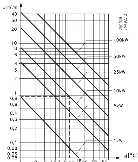
Fig.1 Erwärmung oder Abkühlung mit Wasser.
