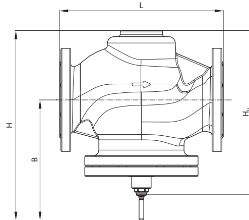
VFG 22(1) DN 65-250
