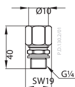
Klemmverbinder
