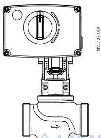
AME 25, AME 35 + Adapter (065Z0311) VRB-2- und VRB-3-Ventile mit Außengewinde (DN 15–50) VRG-2- und VRG-3-Ventile mit Außengewinde (DN 15–50)
