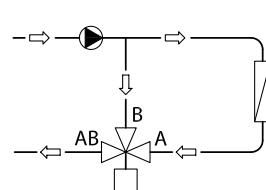
Abb. 3: Mischventil für Verteilanwendungen
