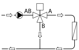
Abb. 4: Verteilventil für Verteilanwendungen
