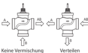
Abb. 1: Misch- oder Verteilanschluss
