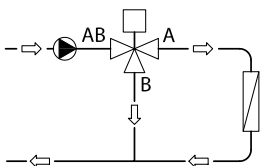
Abb. 4: Verteilventil
