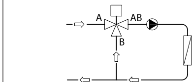
Abb. 2: Mischventil
