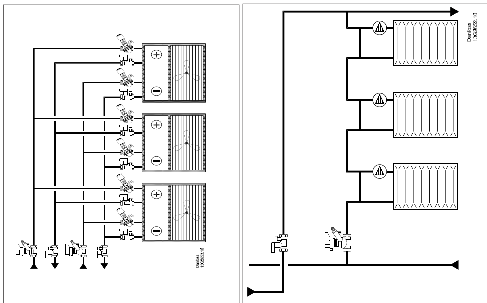
Ventilator-konvektionen (Fan-Coils)
