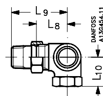
Winkeleck Ventilgehäuse
