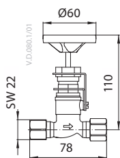
Absperrventil
