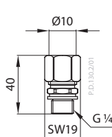
Klemmverbinder
