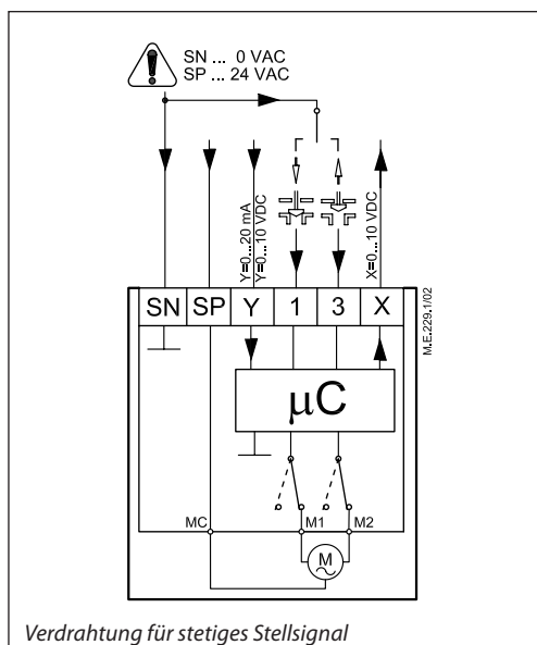
Verdrahtung für stetiges Stellsignal
