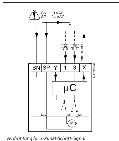
Verdrahtung für 3-Punkt-Schritt-Signal
