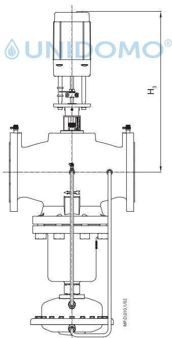
AB-QM DN 125 + AME 55 QM
