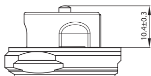
Schließpunkt (Messung) für DN 10–32
