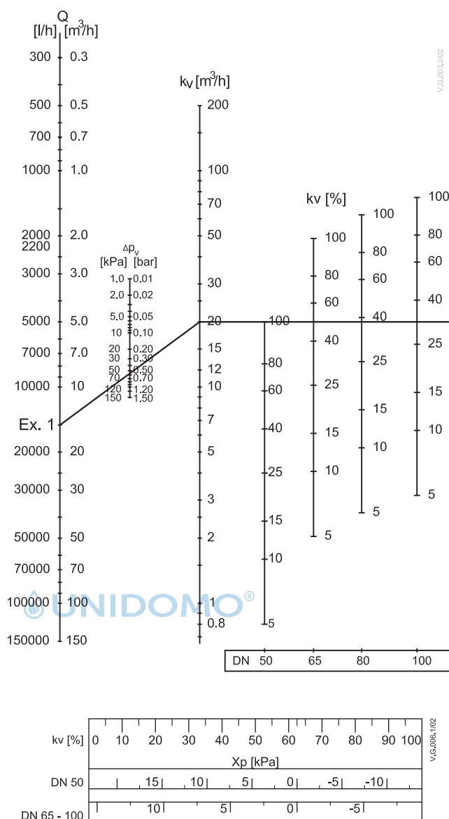
Abb. A - Diagramm zur Dimensionierung von ASV-PV DN 50-100
