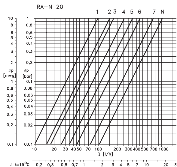
FTC Fühler mit RA-N 20 Ventilgehäuse
