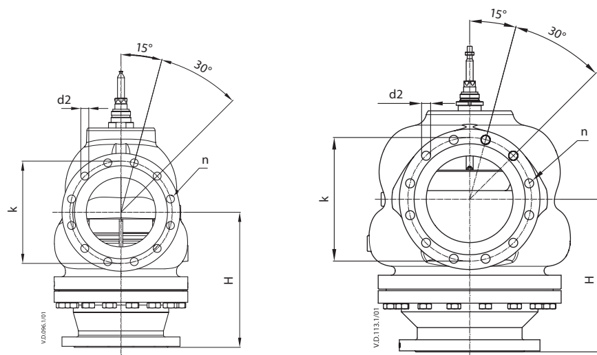
VF 3 (DN 200)
