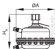
AFQ 2 Druckantrieb
