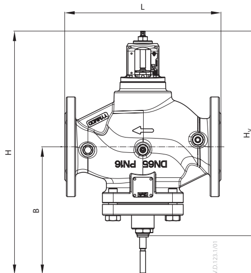
VFQ 22(1) DN 65-250
