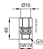
Klemmringverschraubung
