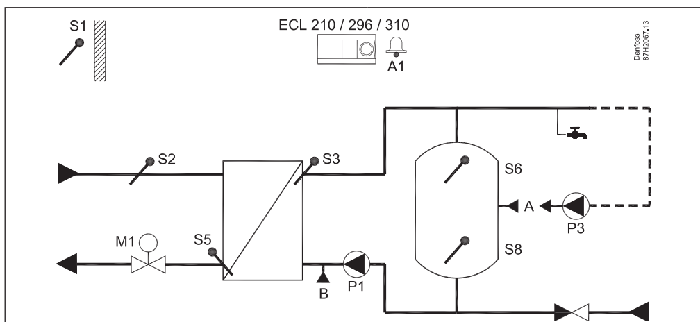
A217.1, Bsp. b: WW-Speicher mit innenliegender Heizschlange
