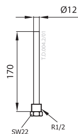
Tauchhülse
