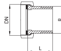
Anschraubenden (Außengewinde)
