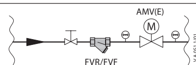
Abb. 2 Mischventil im Rücklauf
