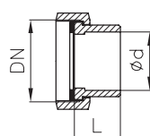
Anschweißenden
