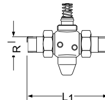
Anschraubendenanschluss
