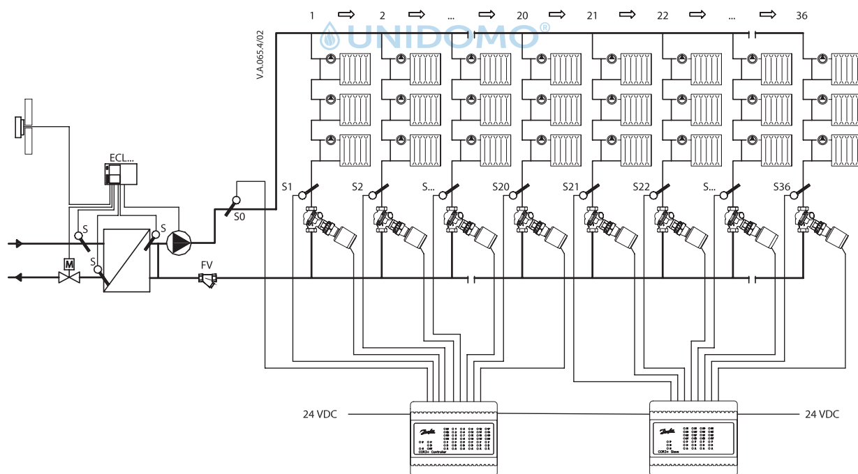
Abb. 2 CCR3+ Regler: Schematische Darstellung mit 36 Strängen
