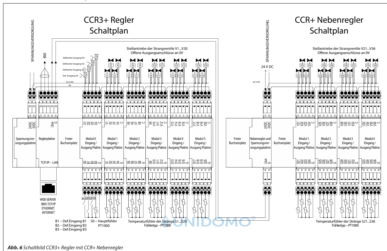
Abb. 6 Schaltbild CCR3+ Regler mit CCR+ Nebenregler
