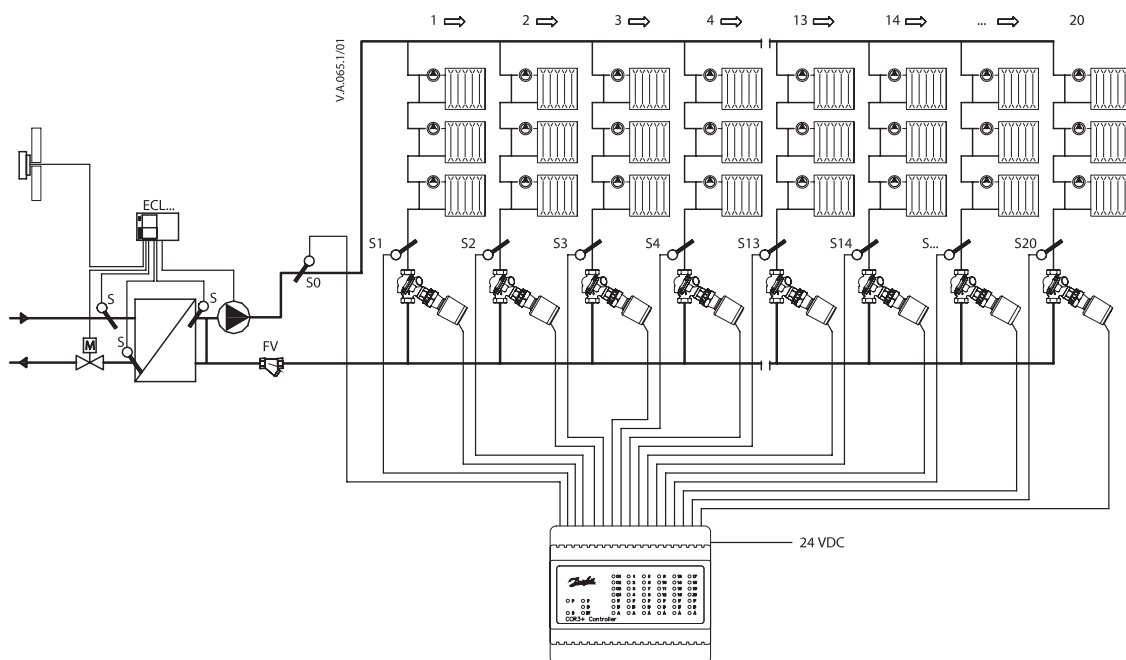
Abb. 1 CCR3+ Regler: Schematische Darstellung mit 20 Strängen
