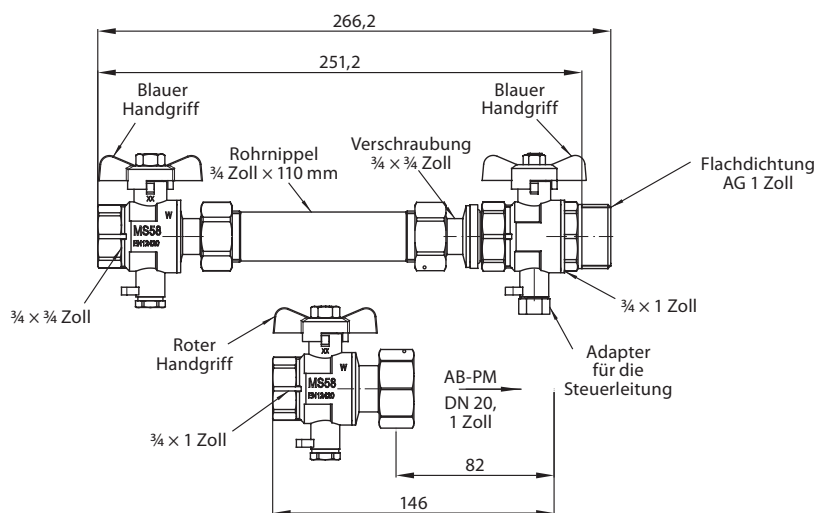
Horizontales Anschluss-Set, DN 20
