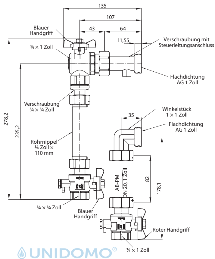
Vertikales Anschluss-Set, DN 20
