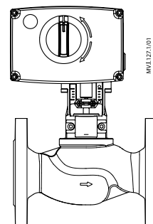
AME 25, AME 35 + Adapter (065Z0311) VF-2- und VF-3-Ventile (DN 15–50) VL-2- und VL-3-Ventile (DN 15–50)
