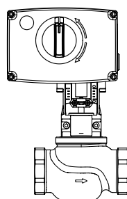
AME 25, AME 35 + Adapter (065Z0311) VRB-2- und VRB-3-Ventile mit Innengewinde (DN 15–50)
