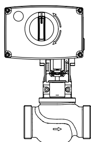
AME 25, AME 35 + Adapter (065Z0311) VRB-2- und VRB-3-Ventile mit Außengewinde (DN 15–50) VRG-2- und VRG-3-Ventile mit Außengewinde (DN 15–50)
