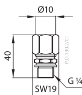
Klemmverbinder
