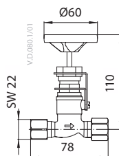
Absperrventil
