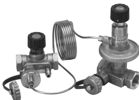
USV-PV / I
