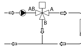
Abb. 4: Verteilventil
