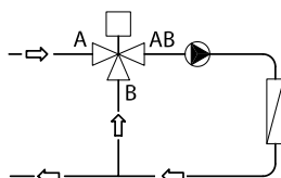
Abb. 2: Mischventil
