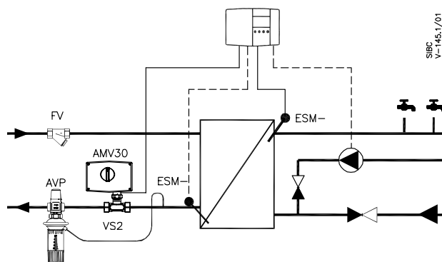
Konstante Temperaturregelung; Wassererwärmungsanlage mit Wärmetauscher
