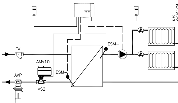
Witterungsgeführte Vorlauftemperaturregelung; Indirekt angeschlossene Hausanlage
