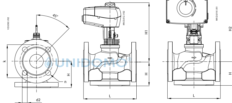
VL 3 (DN 15-80)
