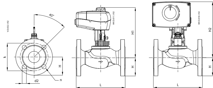
VL 2 (DN 15-80)
